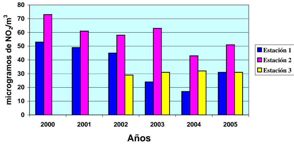
Valores medios anuales de NO 2
